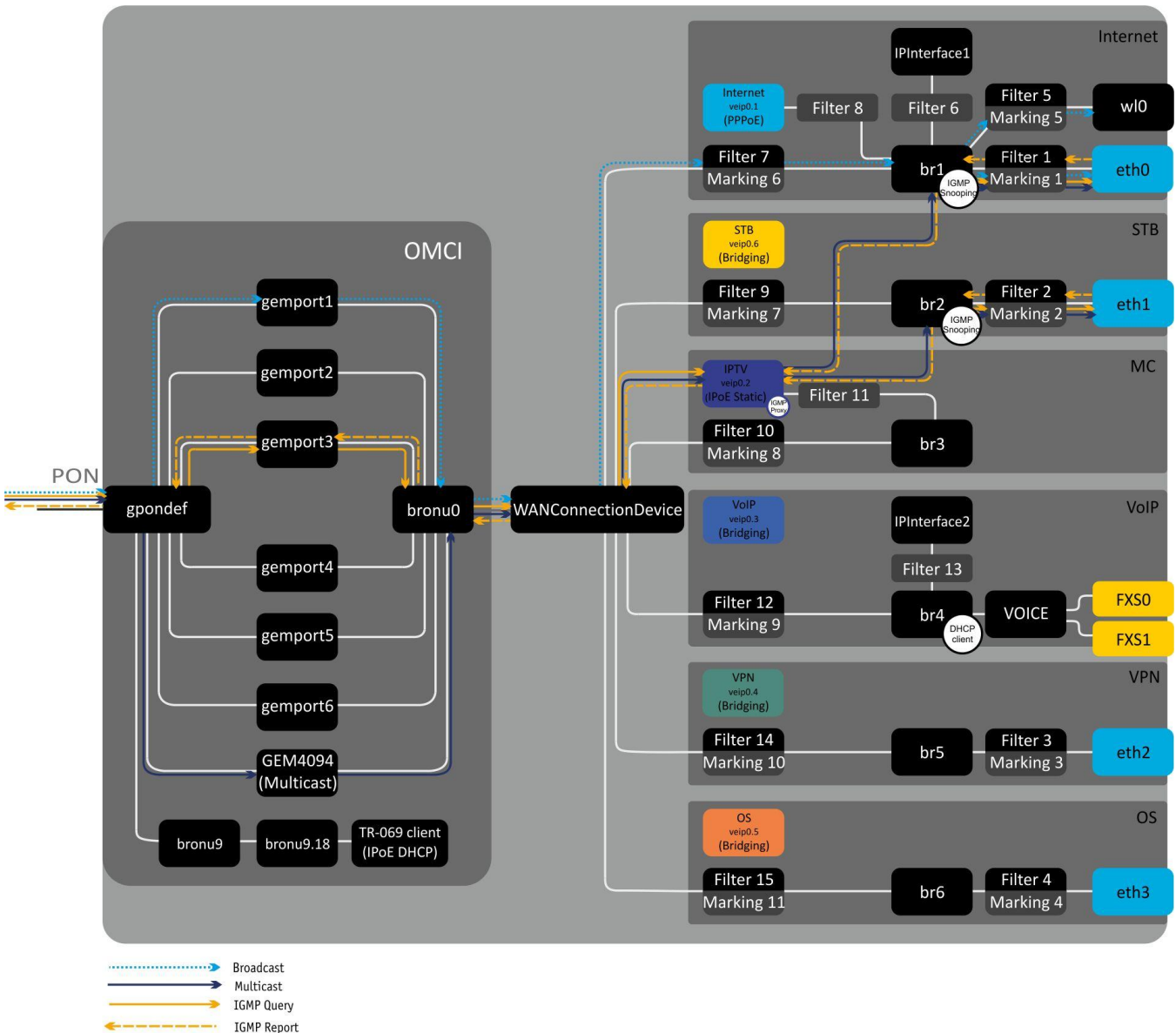
Рисунок 13 – Архитектура устройства, сконфигурированного для предоставления услуг Triple Play по модели 1
