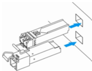
Рисунок 39 – Установка SFP-трансиверов
