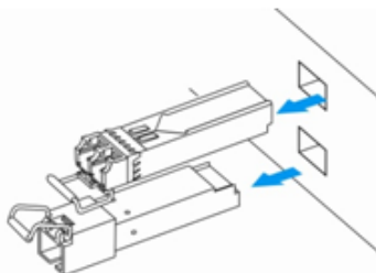
Рисунок 42 – Извлечение SFP-трансиверов
