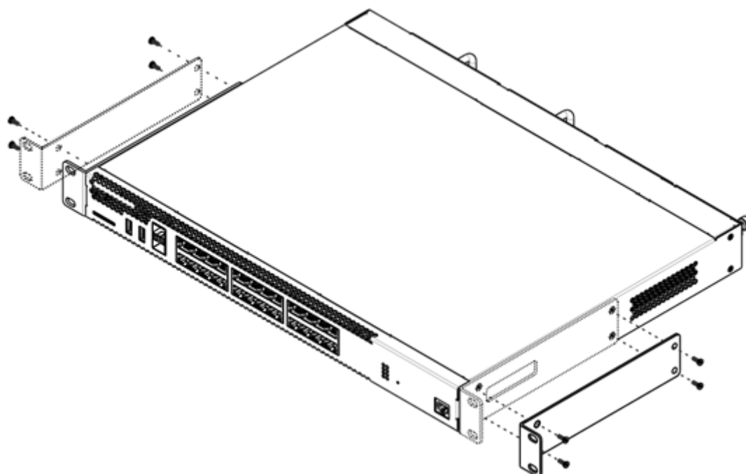
Рисунок 35 – Крепление кронштейнов
