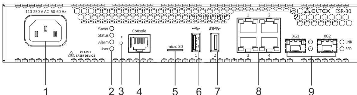
Рисунок 23 – Передняя панель ESR-30
