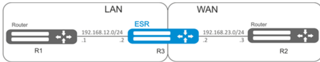
Рисунок 37 – Схема сети
