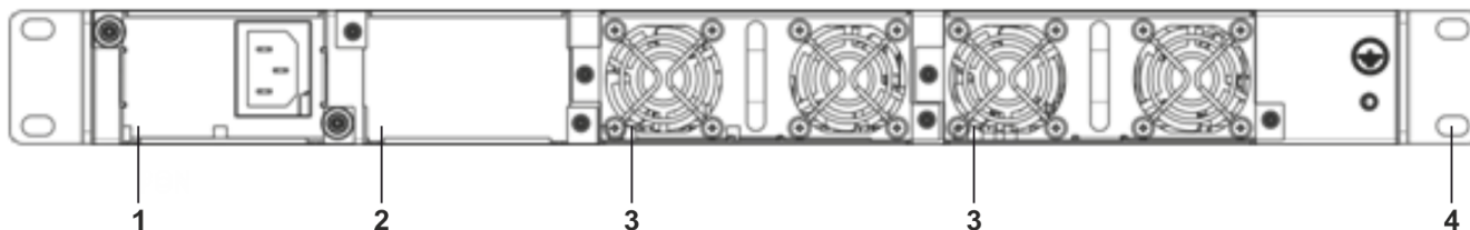
Рисунок 11 – Задняя панель ESR-1000
