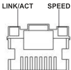
Рисунок 28 – Расположение индикаторов разъема RJ-45
